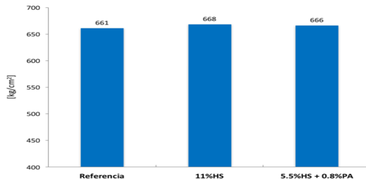
Figura 4. Resistencia a la compresión a 28 días de distintas propuestas de concreto durable.
