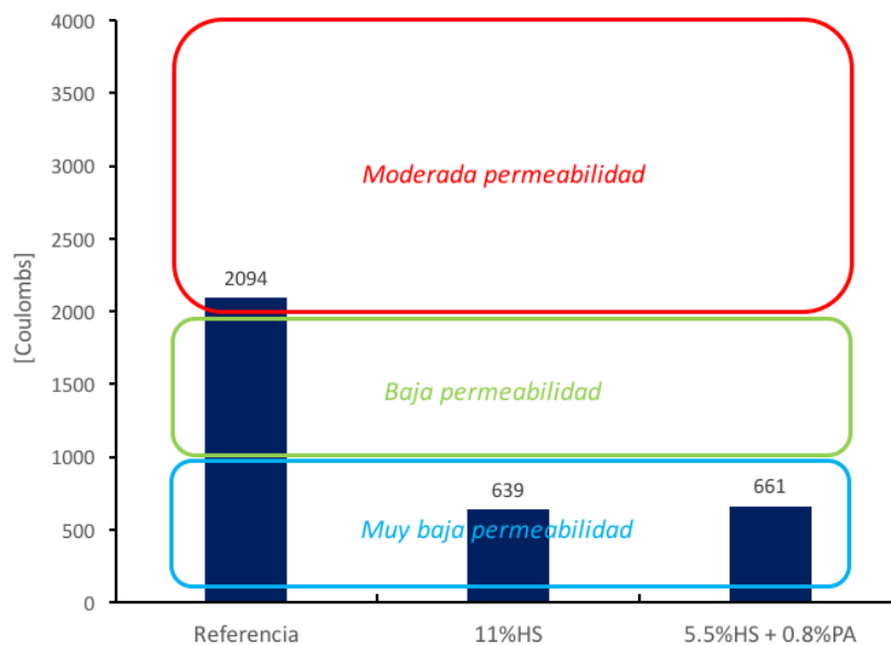
Figura 5. Resistencia a la penetración de iones cloruro a 90 días de acuerdo con ASTM C 1202 para las distintas alternativas de concreto durable.
